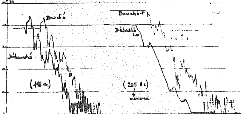
Fig 6 Etude d'un son pur, accordé à la salle d'un vase
