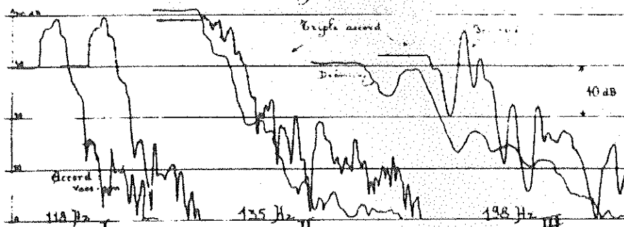
Fig 6 Etude d'un son pur, accordé à la salle d'un vase
